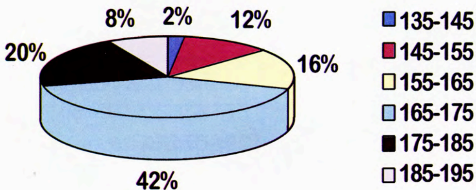
(Σχ. 3.25) Κυκλικό διάγραμμα σχετικών συχνοτήτων.
