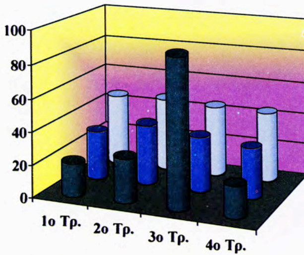
(Σχ. 7.9) Χρονολογικό διάγραμμα με ράβδους
