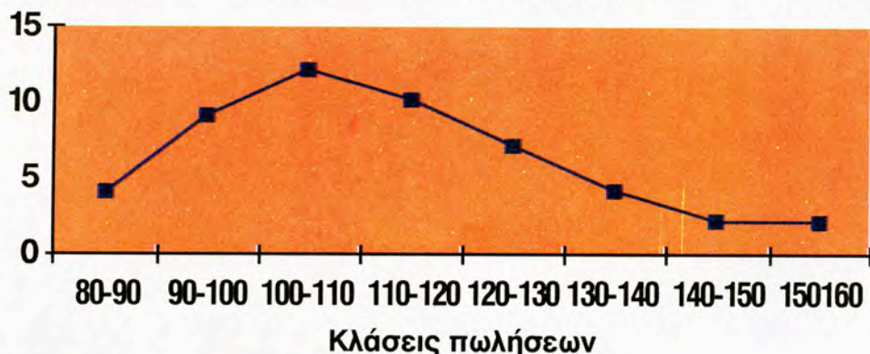
(Σχ.3.9) Πολύγωνο συχνοτήτων.
