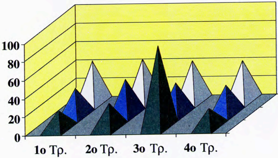
(Σχ. 7.8) Χρονολογικό διάγραμμα με κώνους
