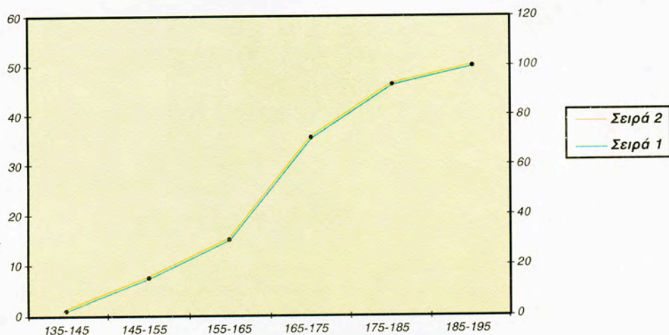
(Σχ. 3.29) Διάγραμμα αθροιστικών συχνοτήτων και σχετικών αθροιστικών συχνοτήτων.
