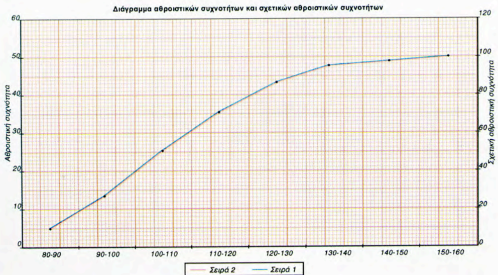
(Σχ.3.11) Διάγραμμα αθροιστικών συχνοτήτων και σχετικών αθροιστικών συχνοτήτων.
