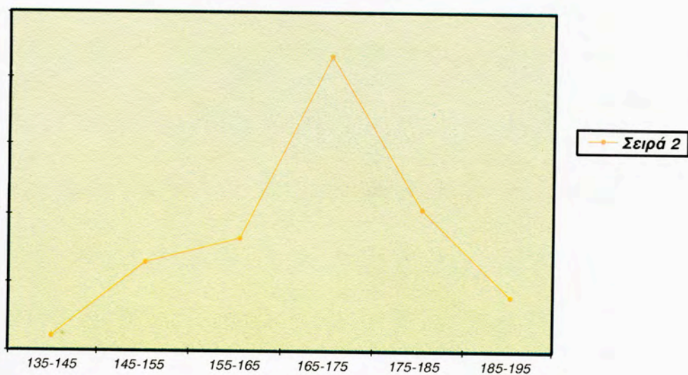
(Σχ. 3.27) Πολύγωνο συχνοτήτων.
