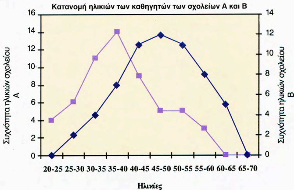
(Σχ. 3.15) Συγκριτικά πολύγωνα συχνοτήτων.
